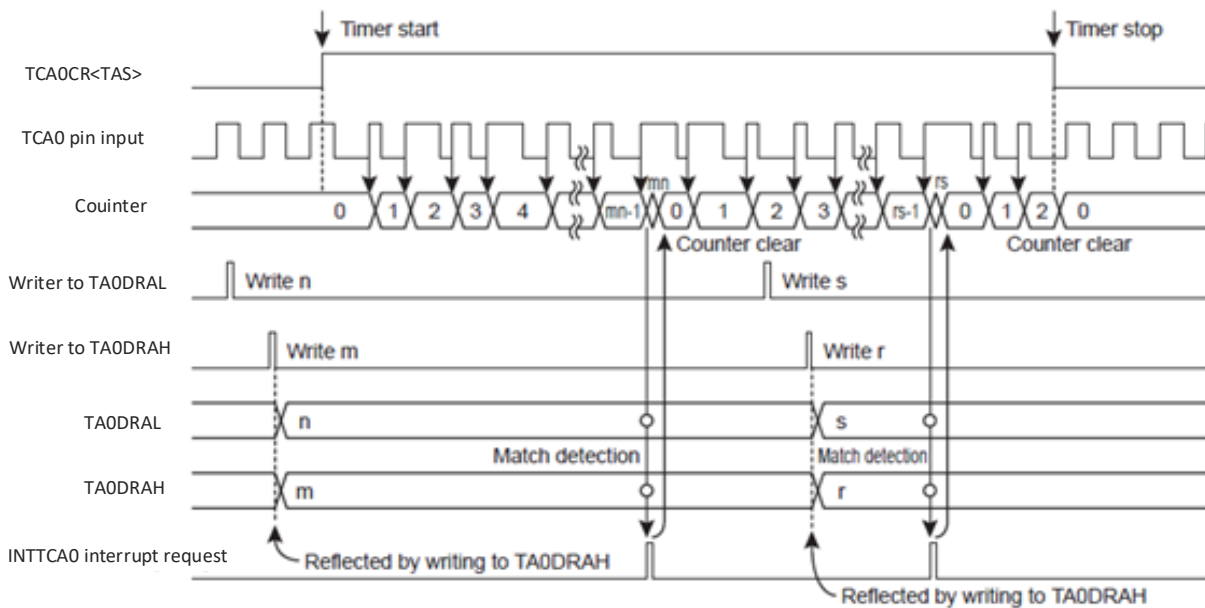
图 12- 15 事件计数器模式时序图(TCA0 为范例)
