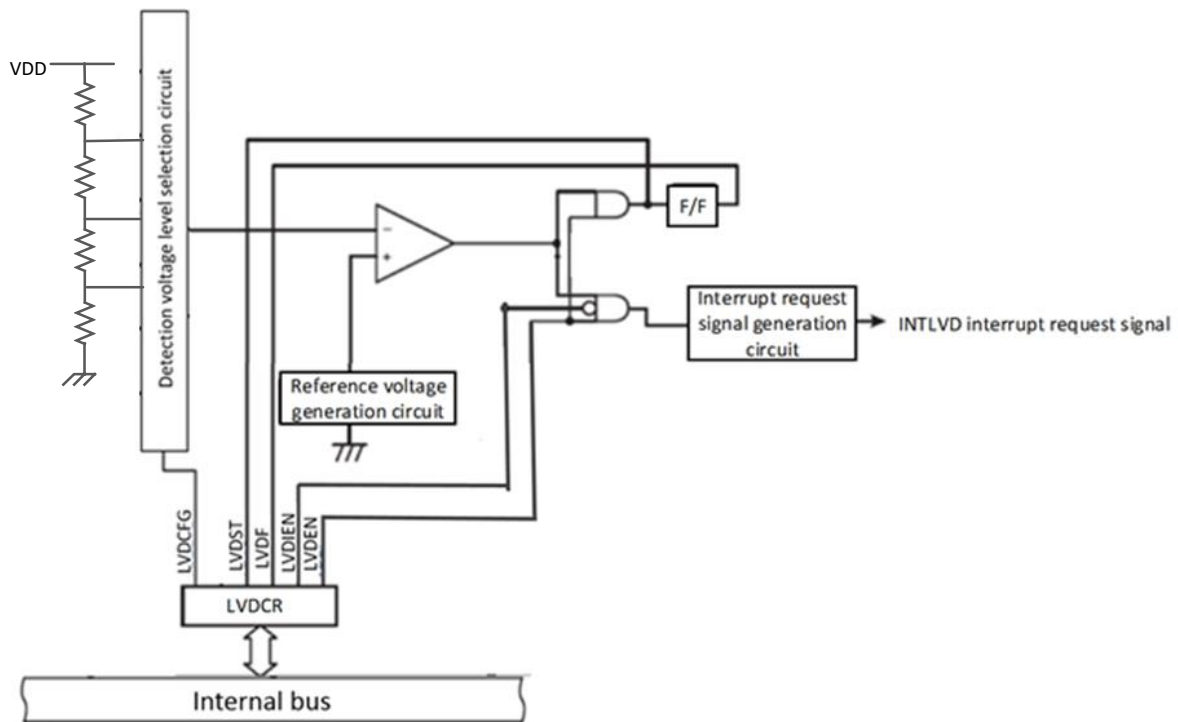
图 5-6 电压检测线路
