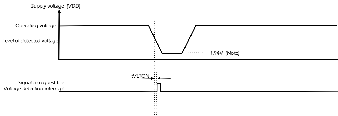
图 2-3 LVD 中断
