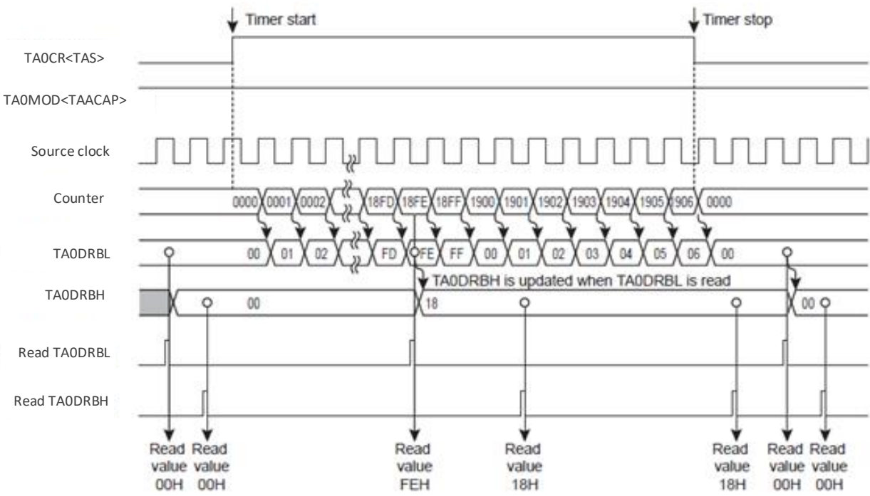
图 12- 13 TCA0 定时器模式范例时序图 (自动抓取)
