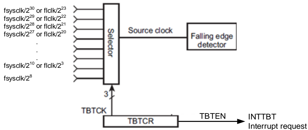
图 12-7 时基定时器架构
