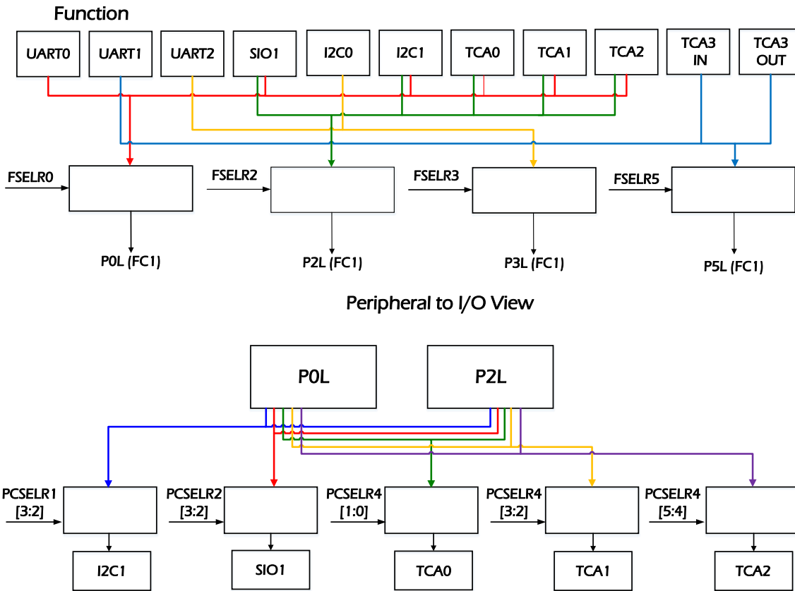
图 11-2 PNIC 架构图
