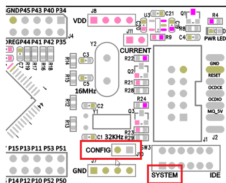
图 A-3 EVB Reset 接地跳帽
