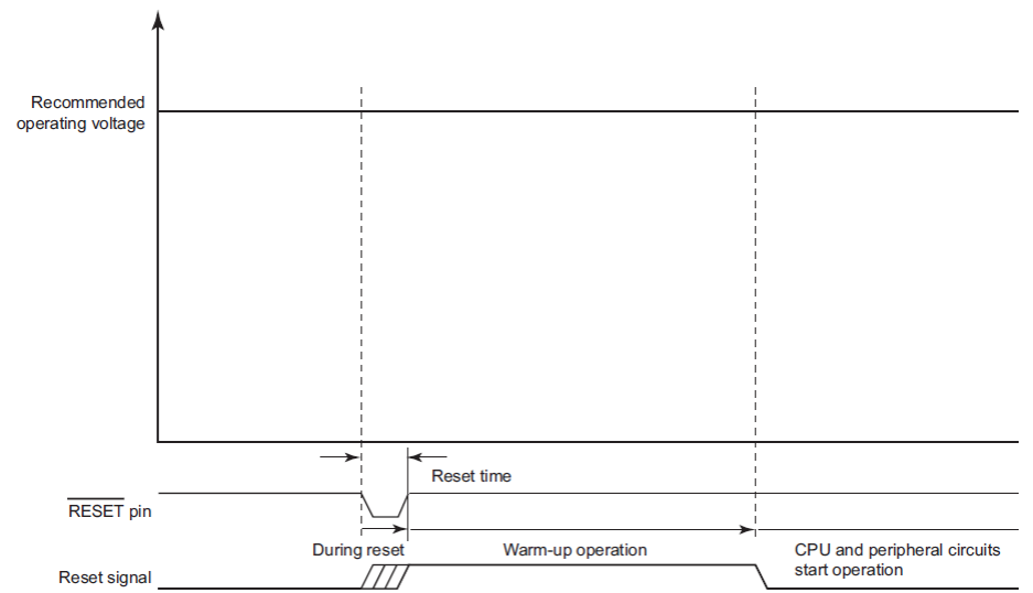
图 5-3 外部复位输入(电压稳定时)
