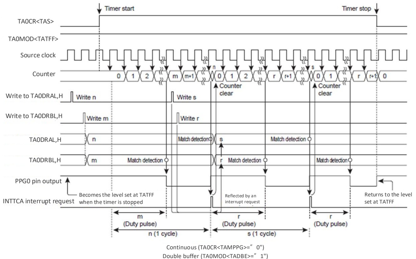
图 12-20 PPG 模式时序图- 连续输出(TCA0 为范例)
