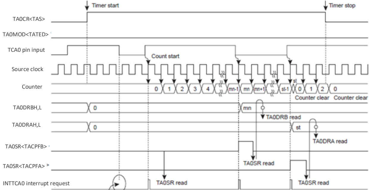
图 12- 17 脉宽测量模式时序图(TCA0 为范例)
