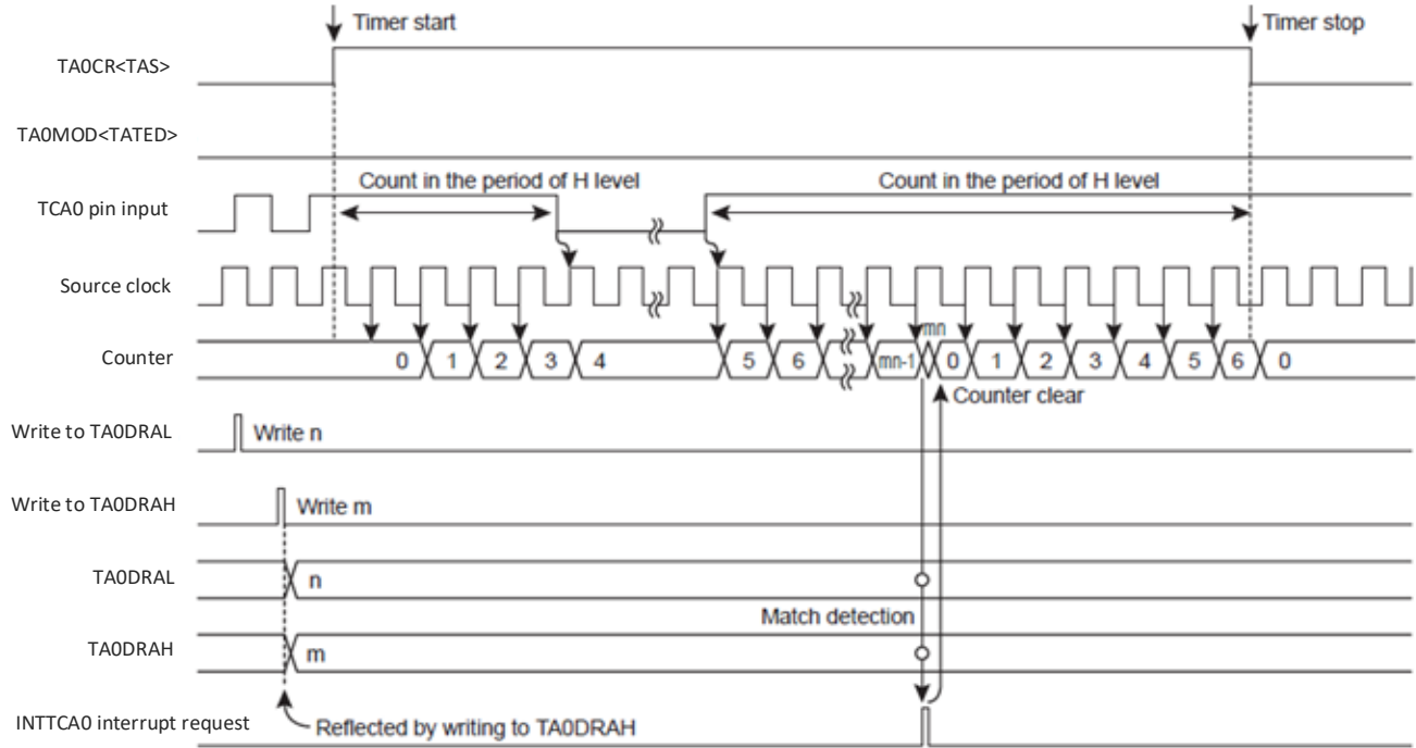
图 12- 16 窗模式时序图(TCA0 为范例)
