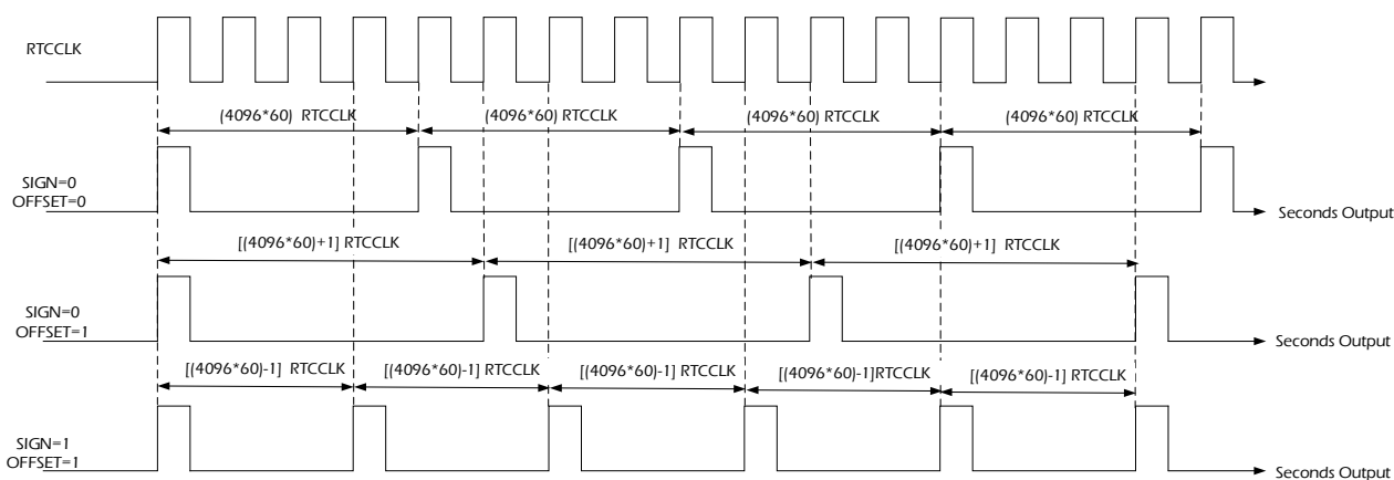
图 12-10 RTC 在 MODE=0 下校正时序范例
