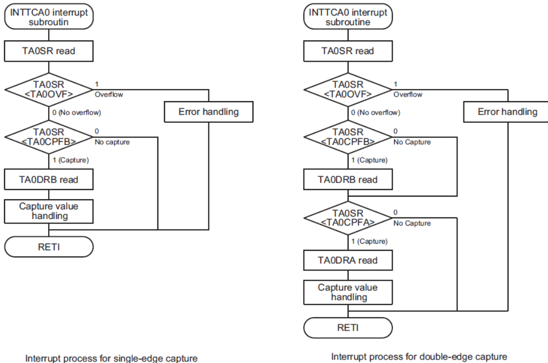
图 12- 18 TCA0 抓取进程范例
