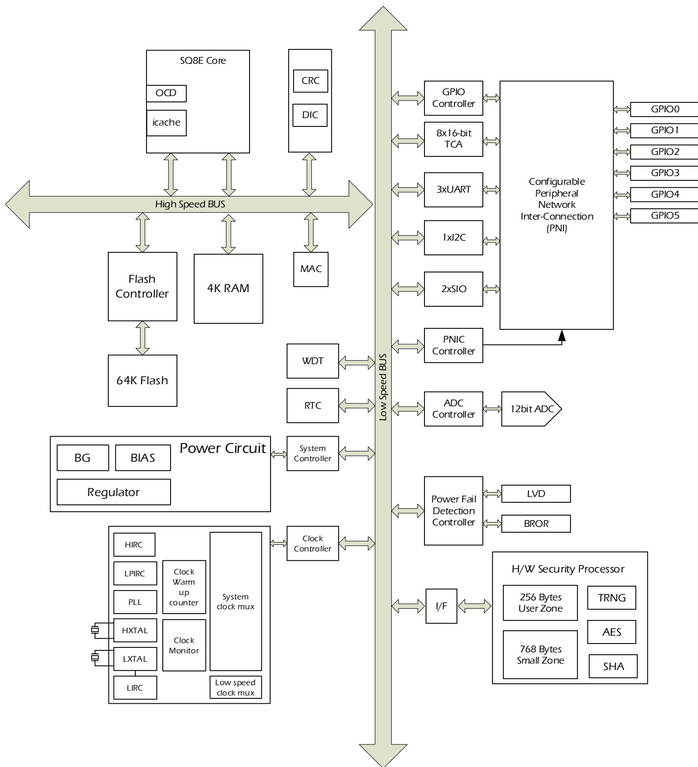
图 1-1 系统模块图
