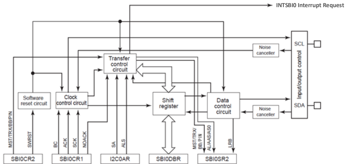
图 14-4 串行总线接口 0 (SBI0)方框图
